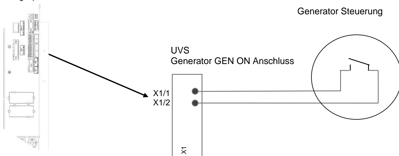
Abb. 1.3: Anschluss des Generator ON Signals
